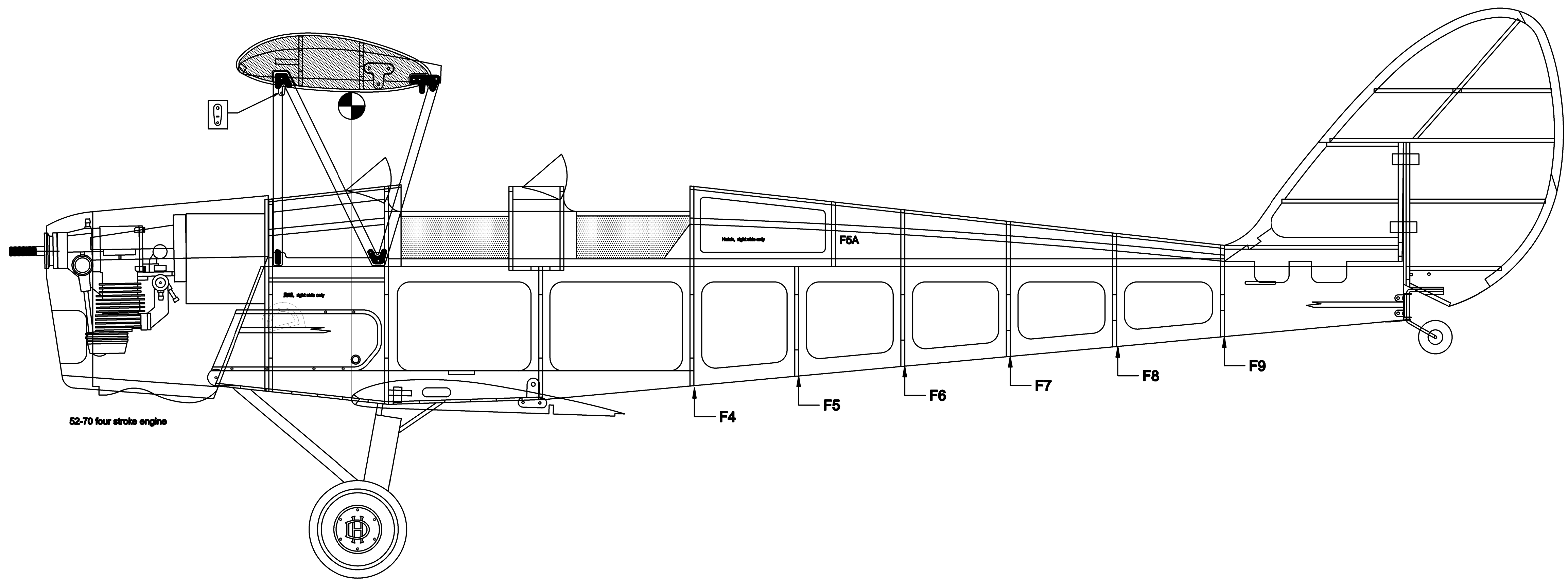
FUSELAGE 1:2
