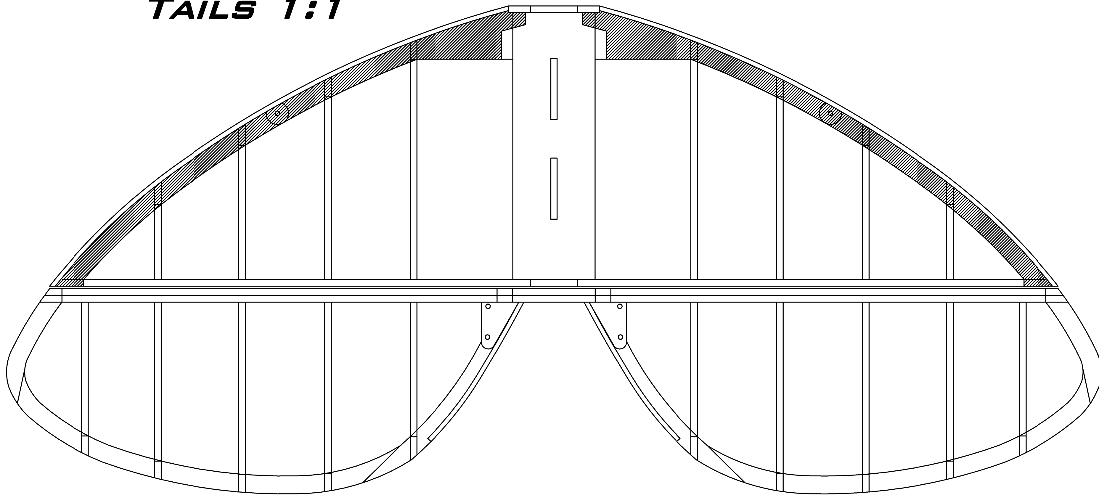
TAILS 1:1
